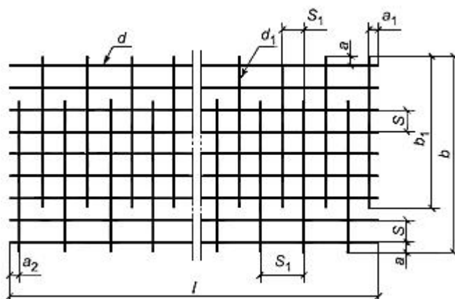
Рисунок 2 - Легкие сетки
